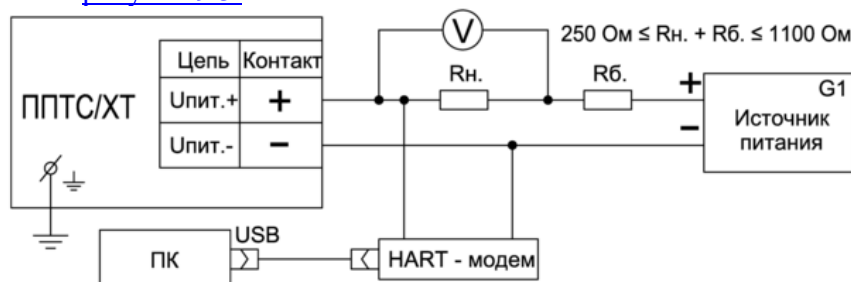
Рисунок 9.3. Схема подключения ППТС/ХТ-PR, ППТС/ХТ-Э и ППТС/ХТ-W к источнику питания G1, сопротивлению нагрузки R_n , вольтметру V и ПК при настройке и измерениях
