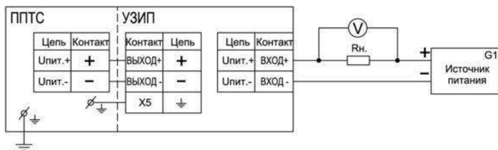
Рисунок 9.7. Схема электрических соединений при подключении ППТС к УЗИП ТЕРМ 002
