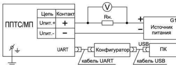
Рисунок 9.1. Схема подключения ППТС/МП к источнику питания G1, сопротивлению нагрузки R_n , вольтметру V и ПК при настройке
