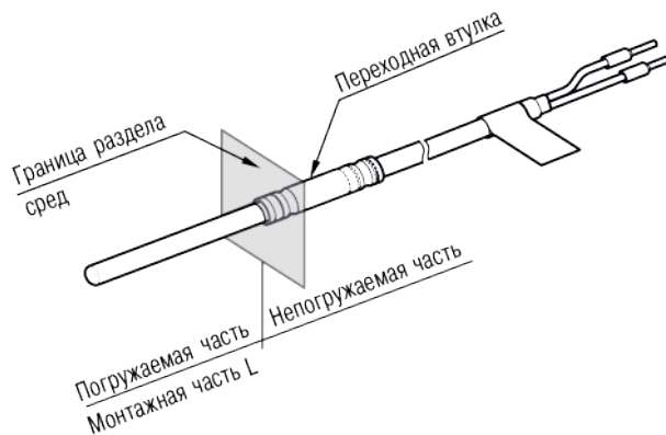
Рисунок 6.1 – Монтаж датчика с кабельным выводом на основе КТМС
