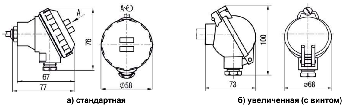
Рисунок Г.2 – Габаритные размеры металлической коммутационной головки
