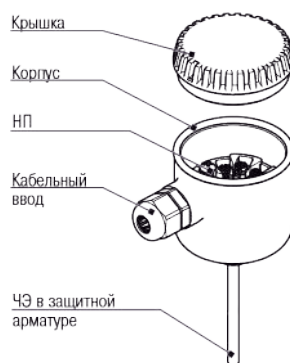
Рисунок 4.1 – Устройство датчика
