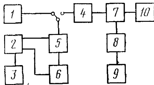
1—источник переменного тока; 2, 8—потенциометры постоянного тока; 3, 9—образцовые меры э. д. с. (нормальный элемент); 4—переключатель направления постоянного тока; 5—эталонный или образцовый преобразователь; 6—поверяемый прибор; 7—образцовая мера сопротивления; 10—источник постоянного тока
