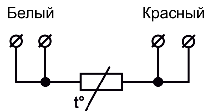
Рисунок Д.3 – Четырехпроводная схема внутренних соединений проводов с одним ЧЭ
