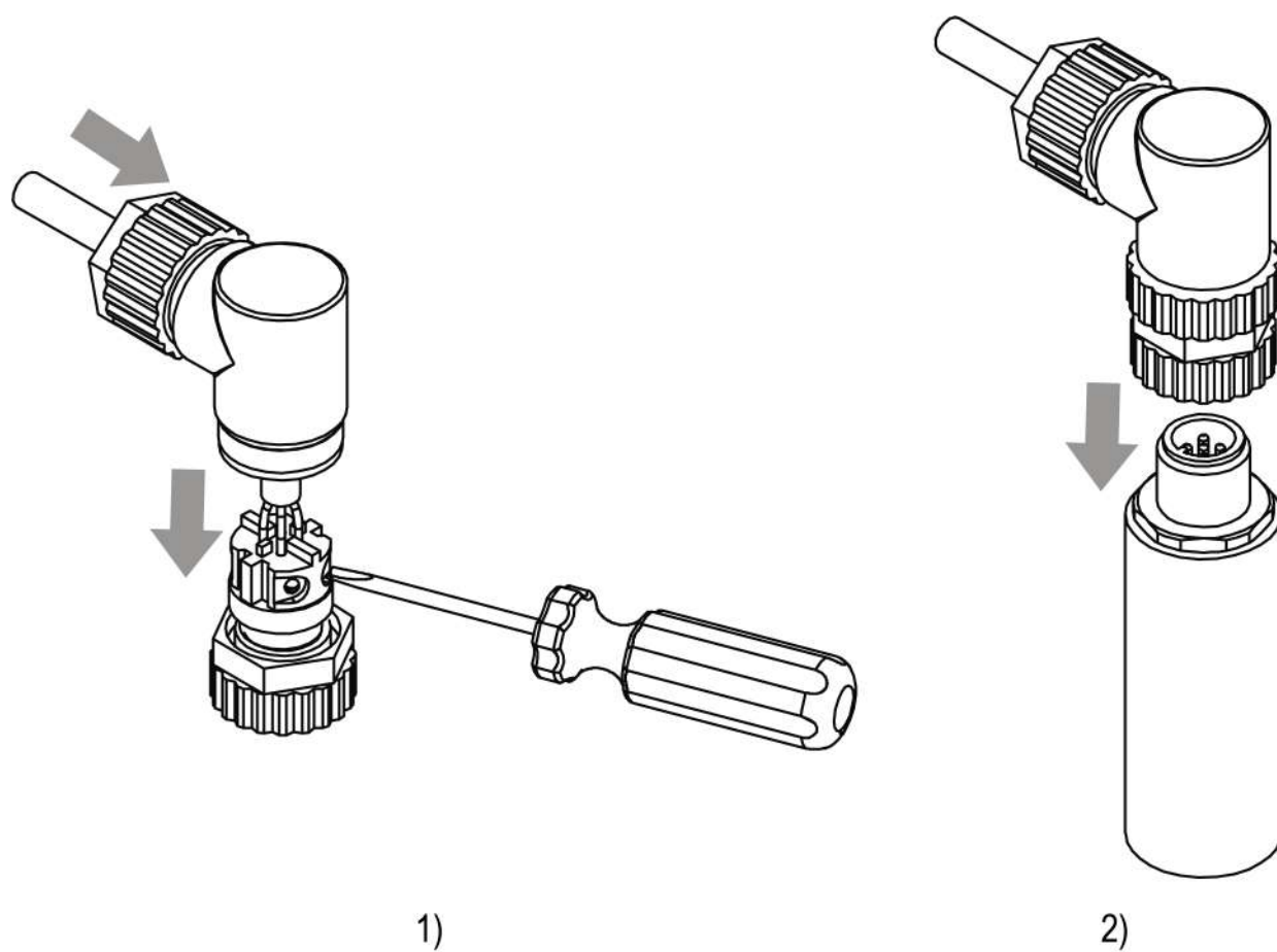
Рисунок 5.2 – Монтаж проводов
